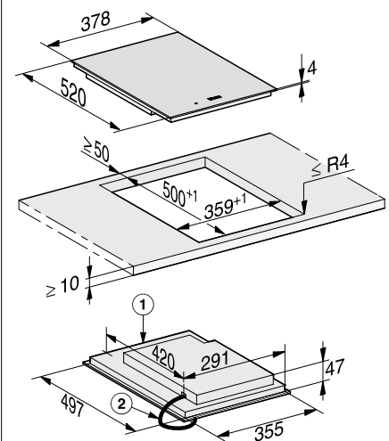
aufliegender Einbau
