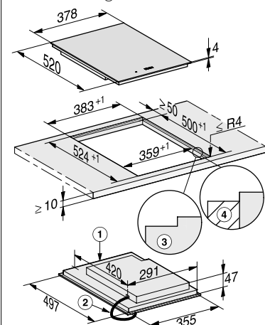
flächenbündiger Einbau
